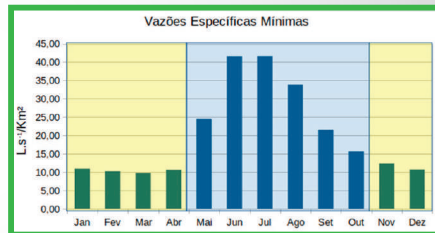
Vazões específicas mínimas mensais médias ao longo do ano, das estações utilizadas neste estudo. O campo amarelo marca o período vazante e o campo azul o período de cheias ("ano hídrico").
